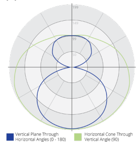
Snag Long 4000K Dimmable
