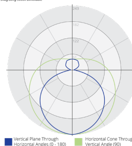
Snag Long 3000K Dimmable
